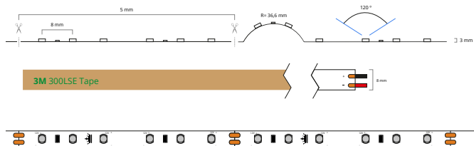
IP20 24V
